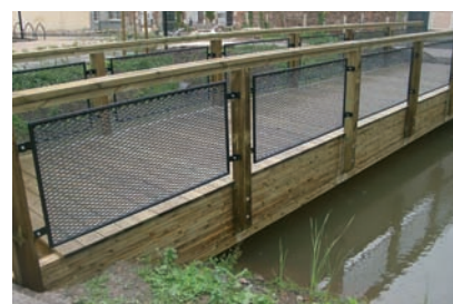
Passerelle cintrée lamellé-collé en pin Garde-corps mixte : pin et métal déployé thermo-laqué
